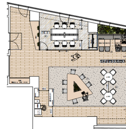
いちごレイアウトオフィス(平面図)
